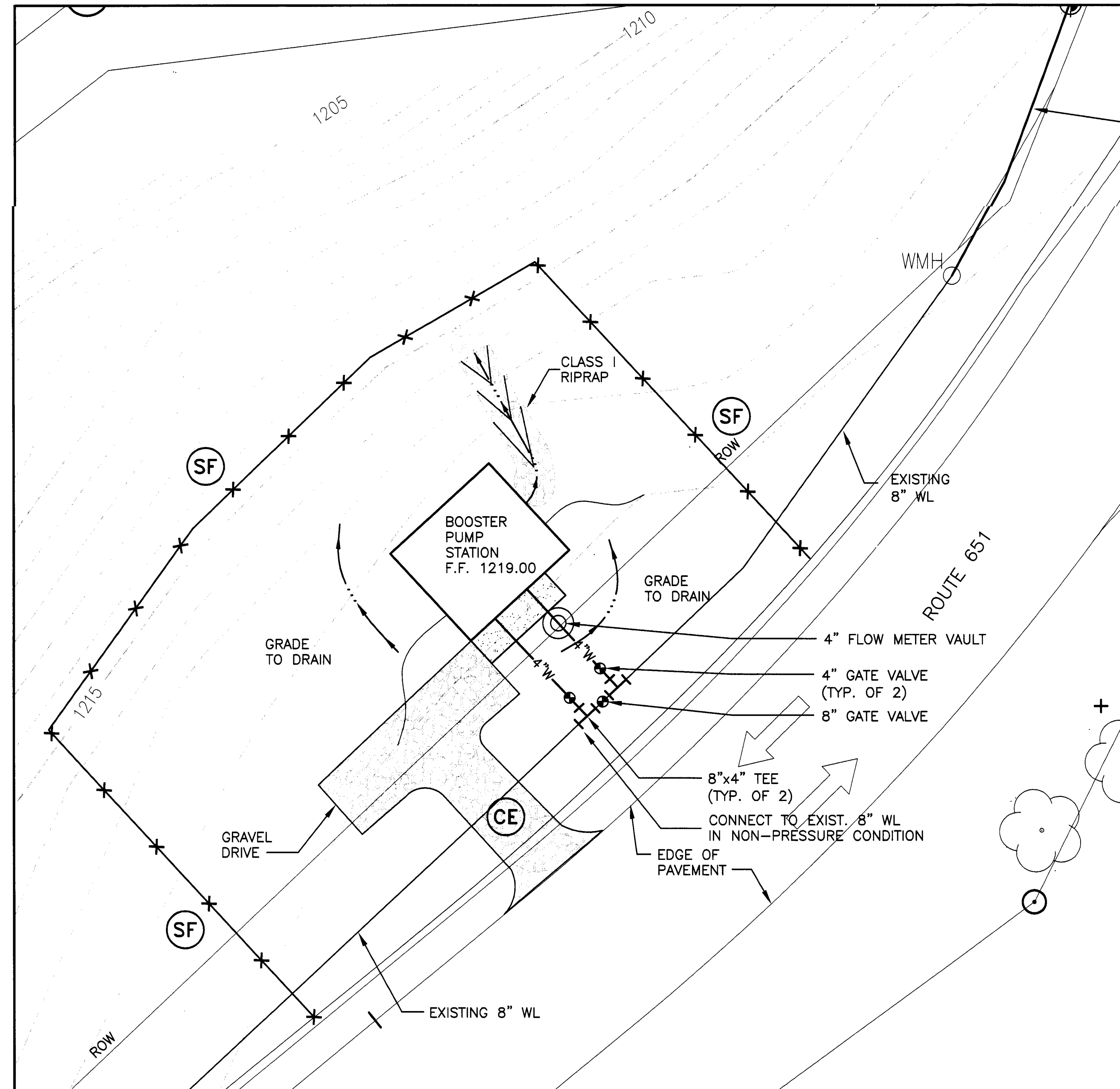
SITE PLAN SCALE: 1" = 10'
