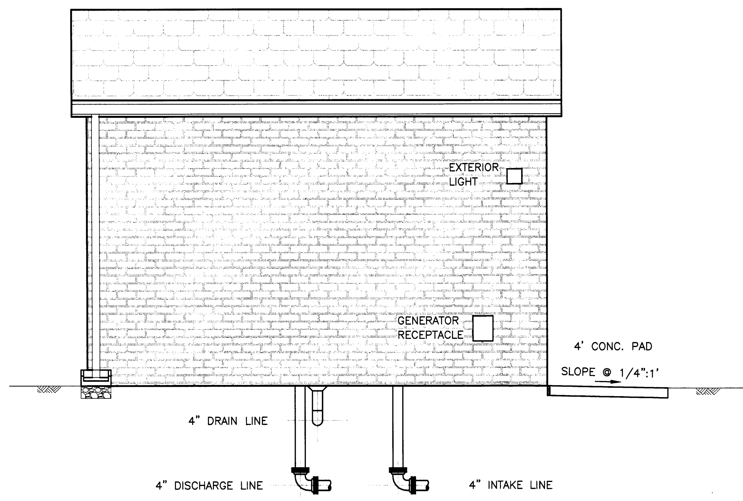
WEST ELEVATION SCALE: 1/2" = 1'-0"
