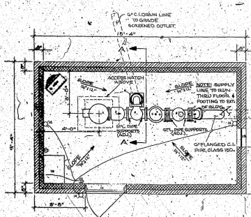
PLAN SCALE 1/4\"/>
