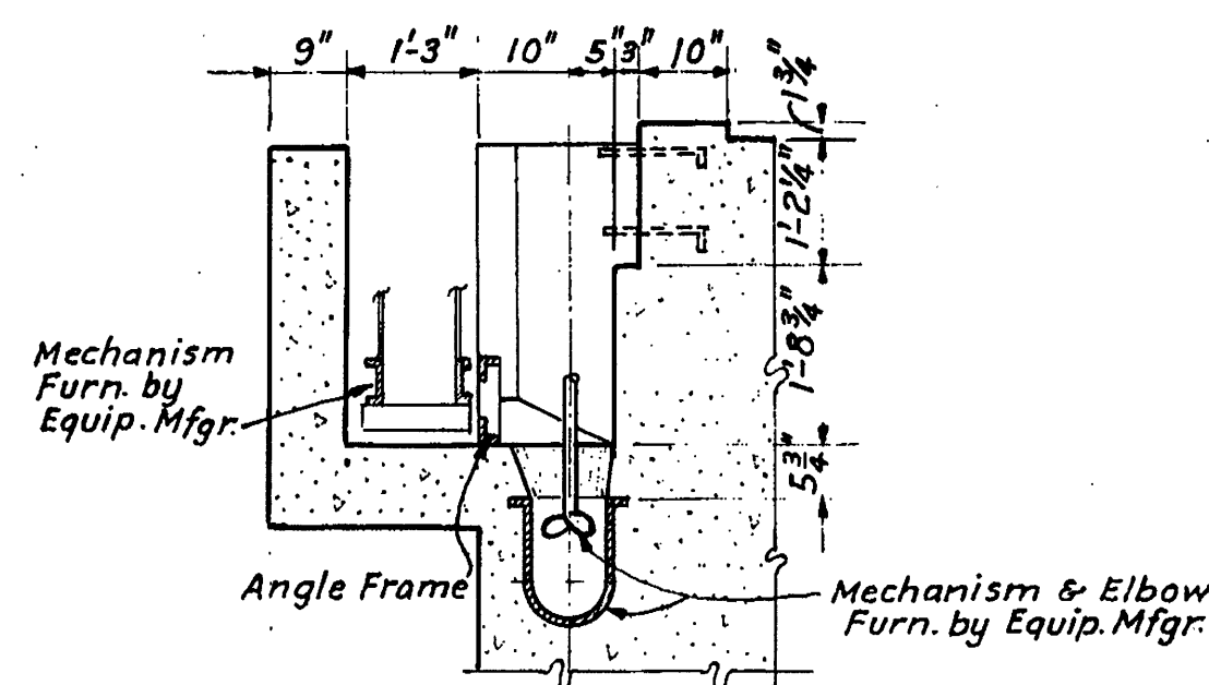
SECTION I-I Scale: 1/2"=1'-0"
