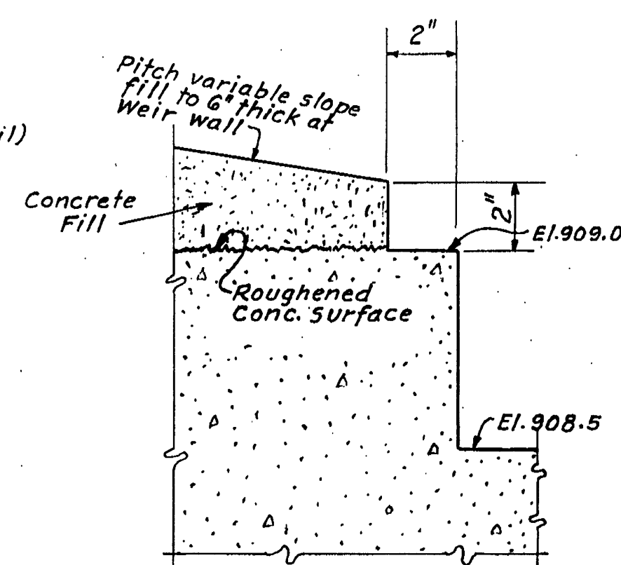
SECTION X-X Scale: 3"=1'-0"
