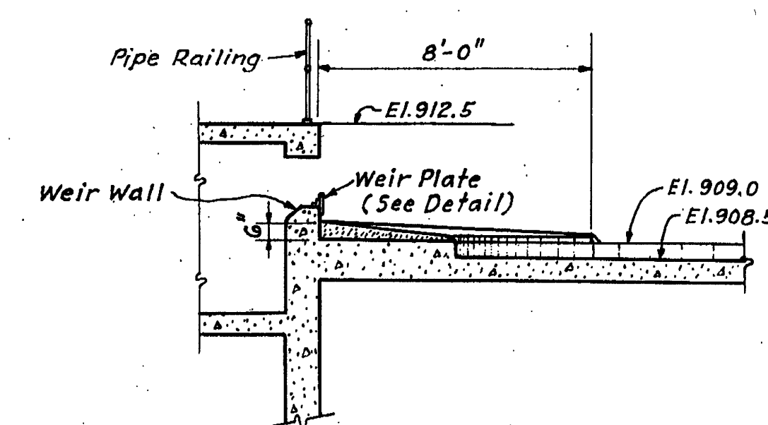
SECTION P-P Scale: 1/2"=1'-0"
