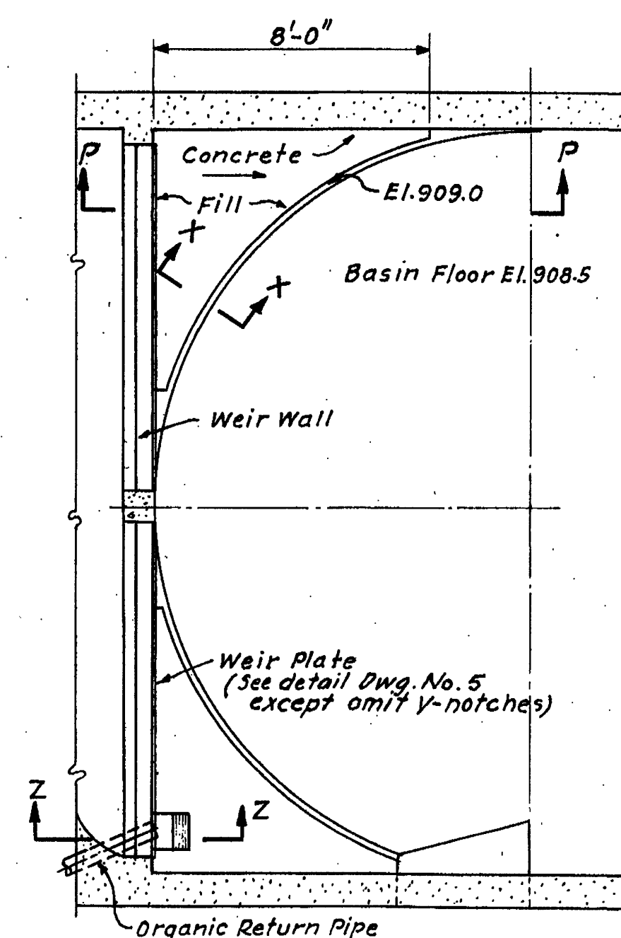
PLAN Scale: 1/2"=1'-0"
