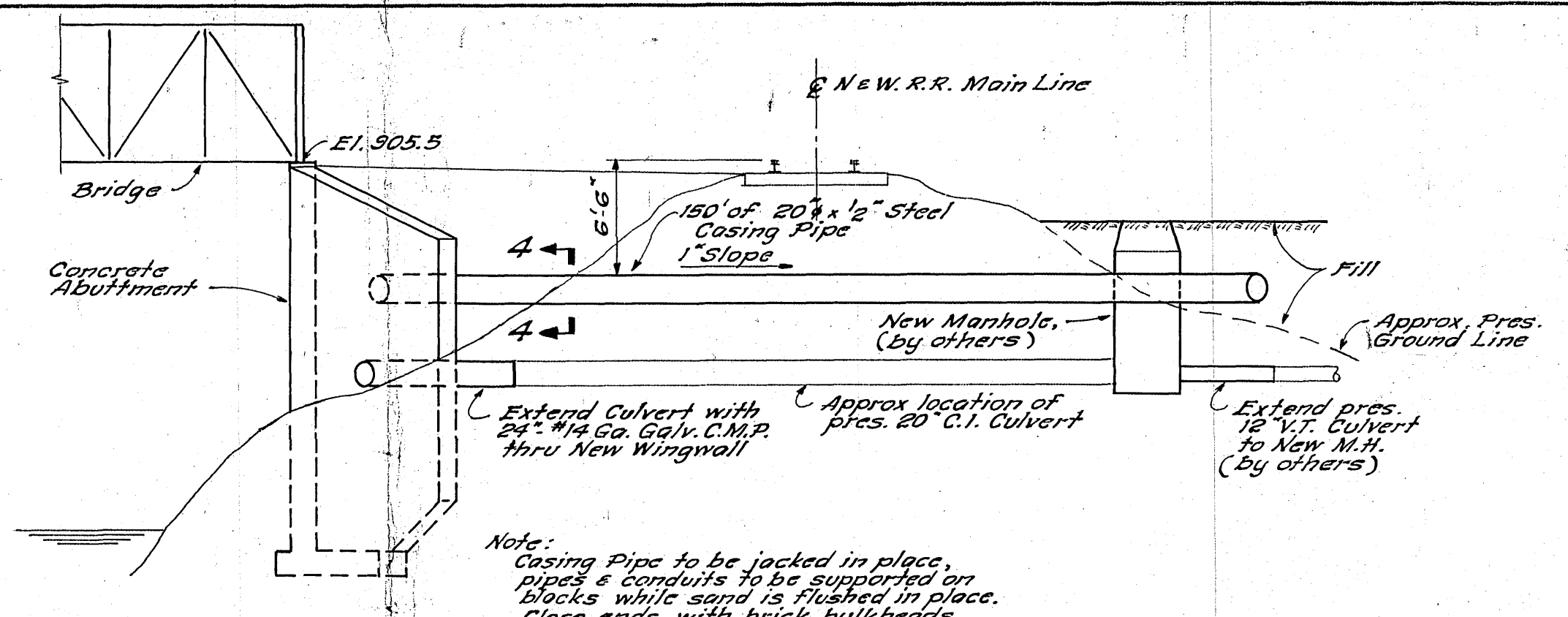
SECTION 3-3 Scale: 1/8" = 1'-0"
