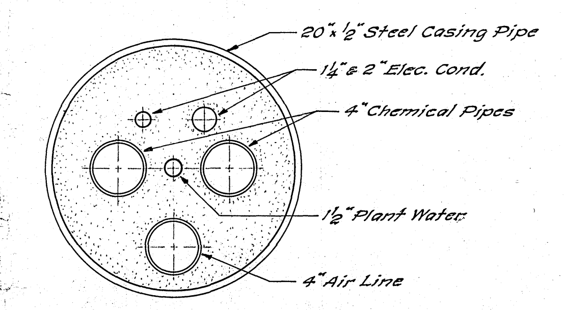
SECTION 4-4 Scale: 1/2" = 1'-0"
