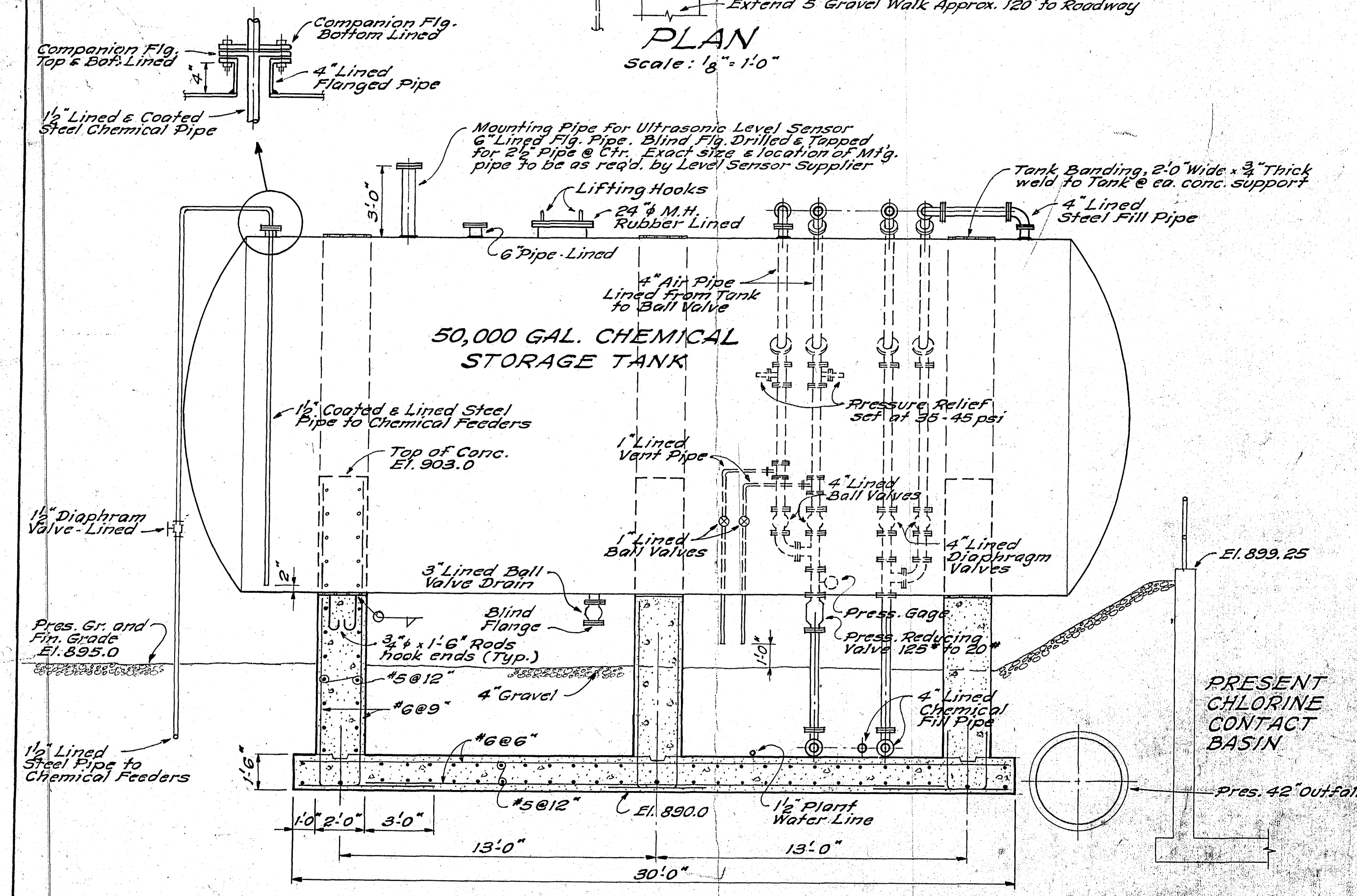
SECTION 1-1 Scale: 1/4" = 1'-0"
