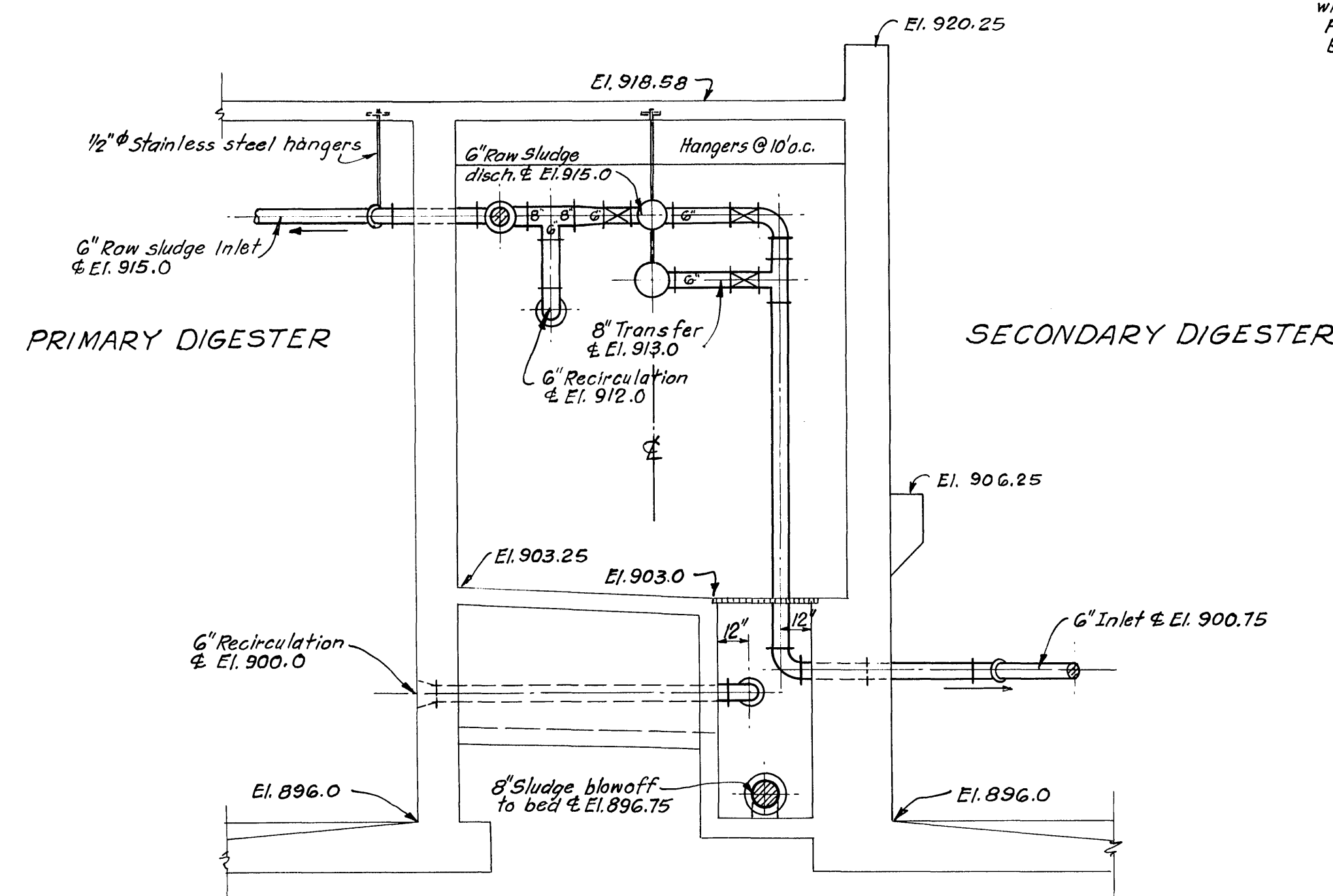
SECTION Q-Q Scale: 1/4" = 1'-0"
