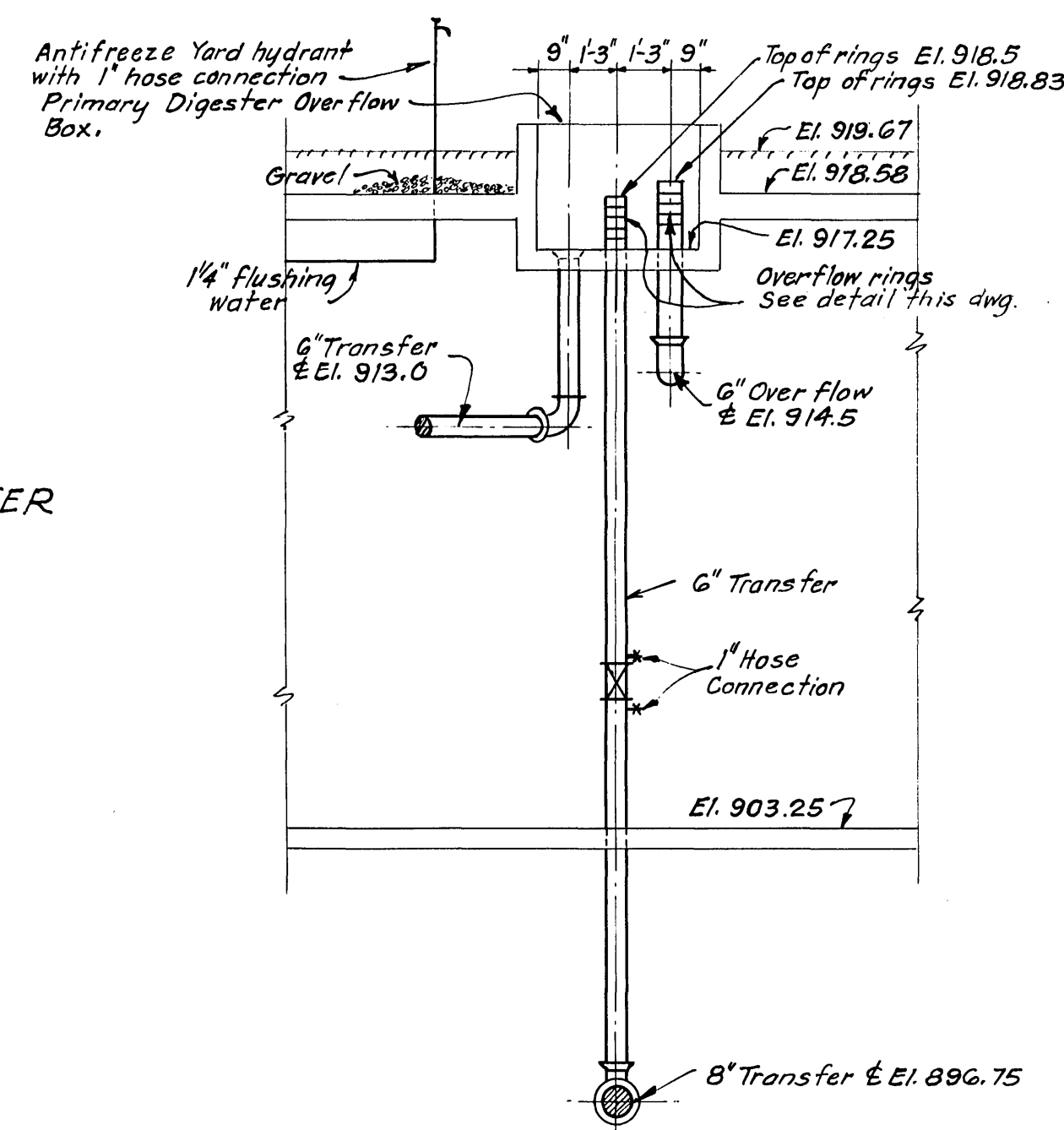
SECTION R-R Scale: 1/4" = 1'-0"
