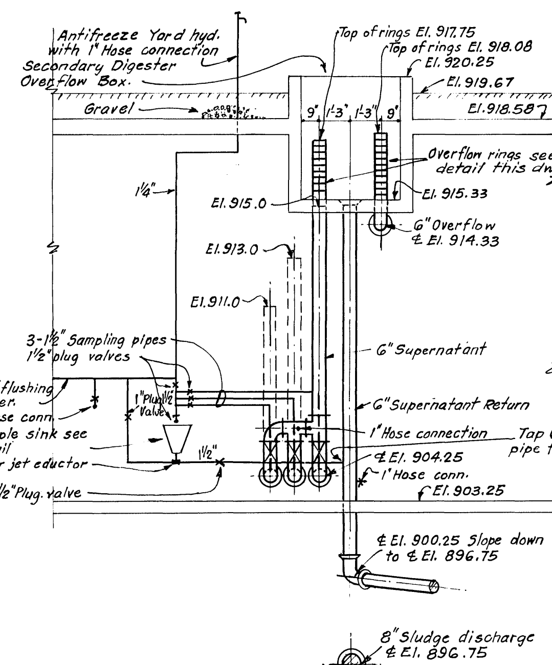
SECTION S-S Scale: 1/4" = 1'-0"
