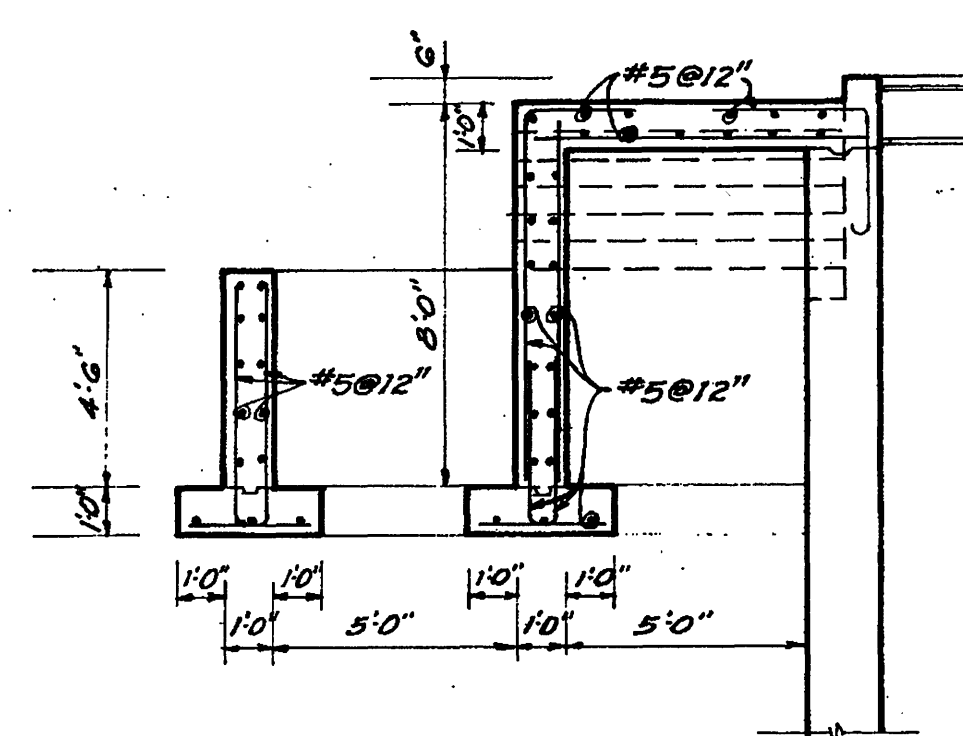
SECTION L 18-19 Scale: 1/4"=1'-0"
