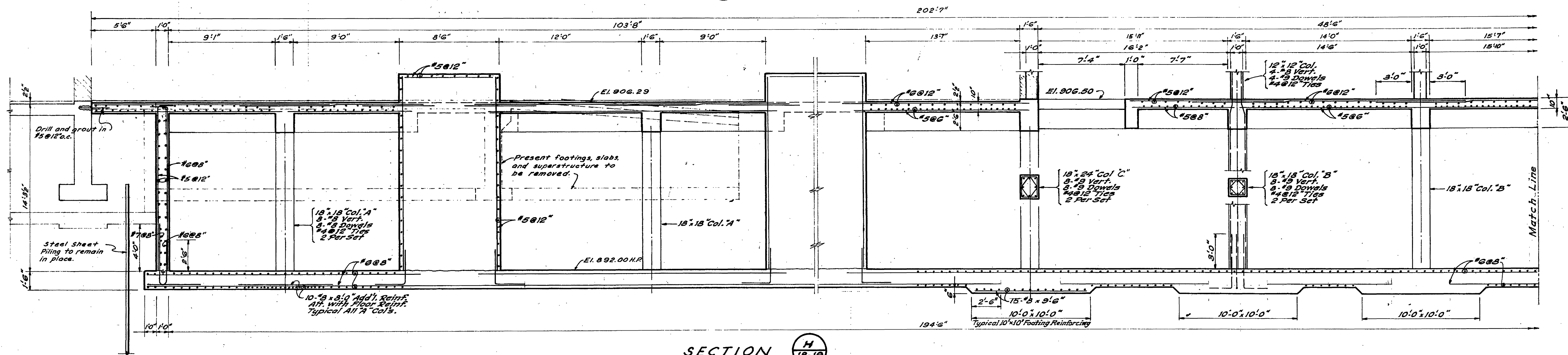
SECTION G 18-19 Scale: 1/4"=1'-0"
