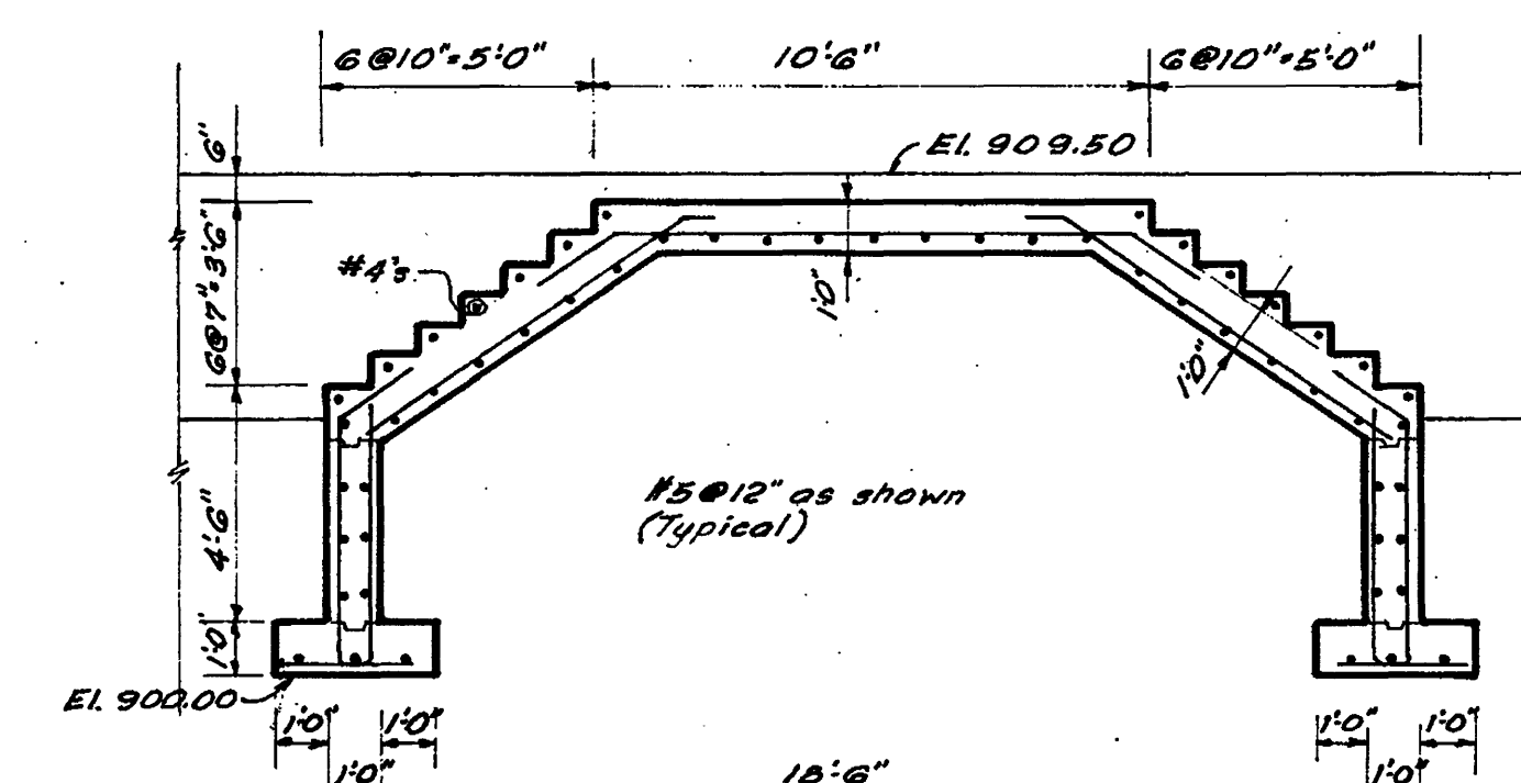
SECTION M 18-19 Scale: 1/4"=1'-0"
