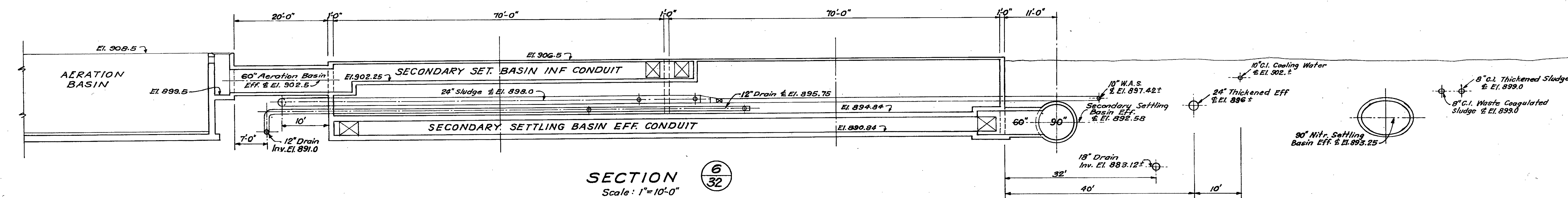
SECTION 5 Scale: 1"=10'-0"
