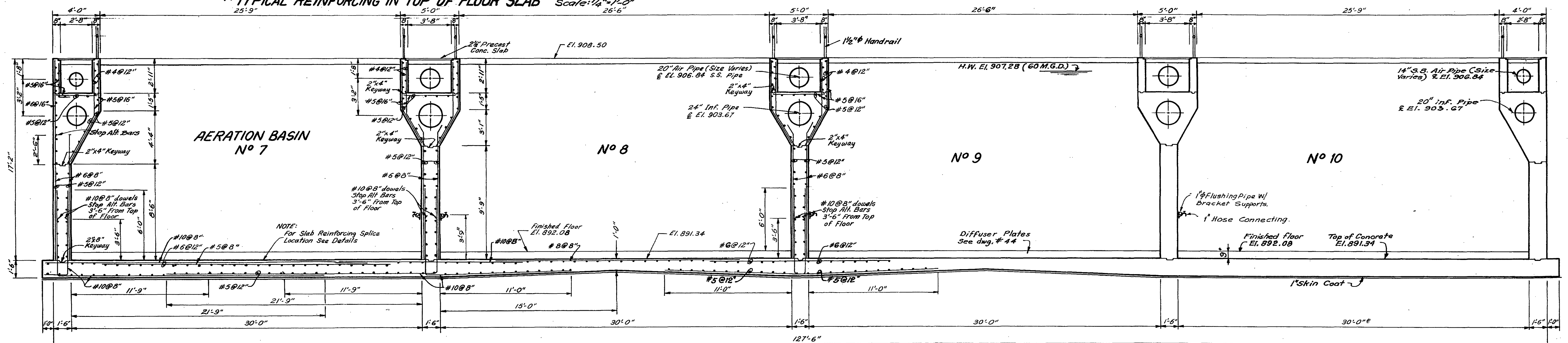
SECTION 8/35 Scale: 1/4" = 1'-0"
