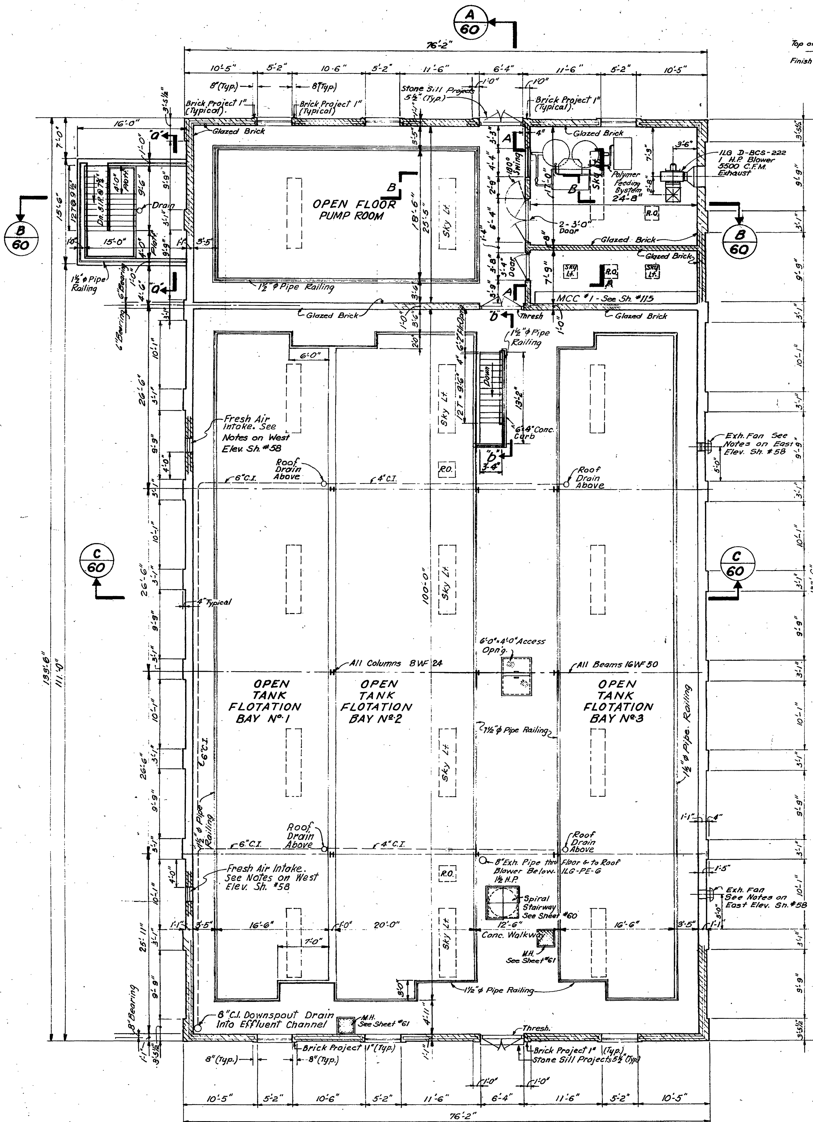
FLOOR PLAN SCALE: 1/8" = 1'-0"
