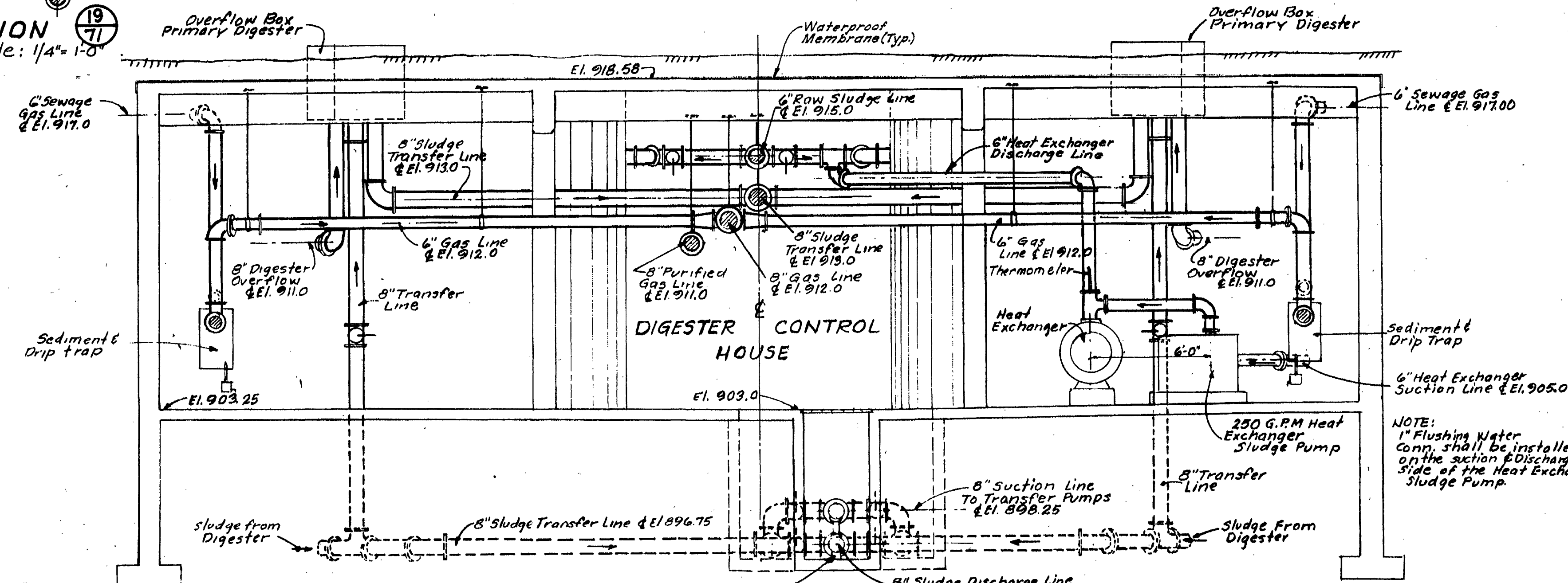
SECTION 21 Scale: 1/4" = 1'-0"
