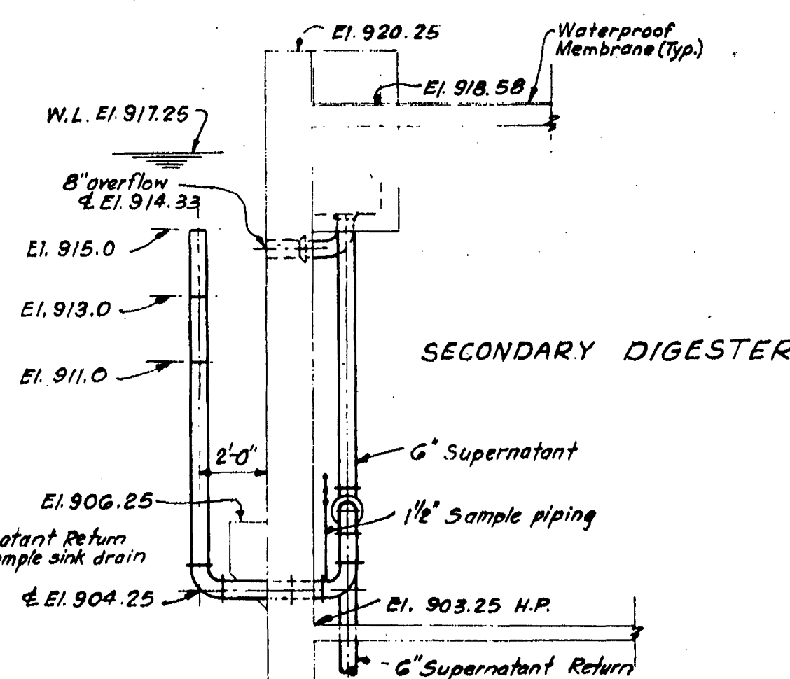
SECTION 20 Scale: 1/4" = 1'-0"
