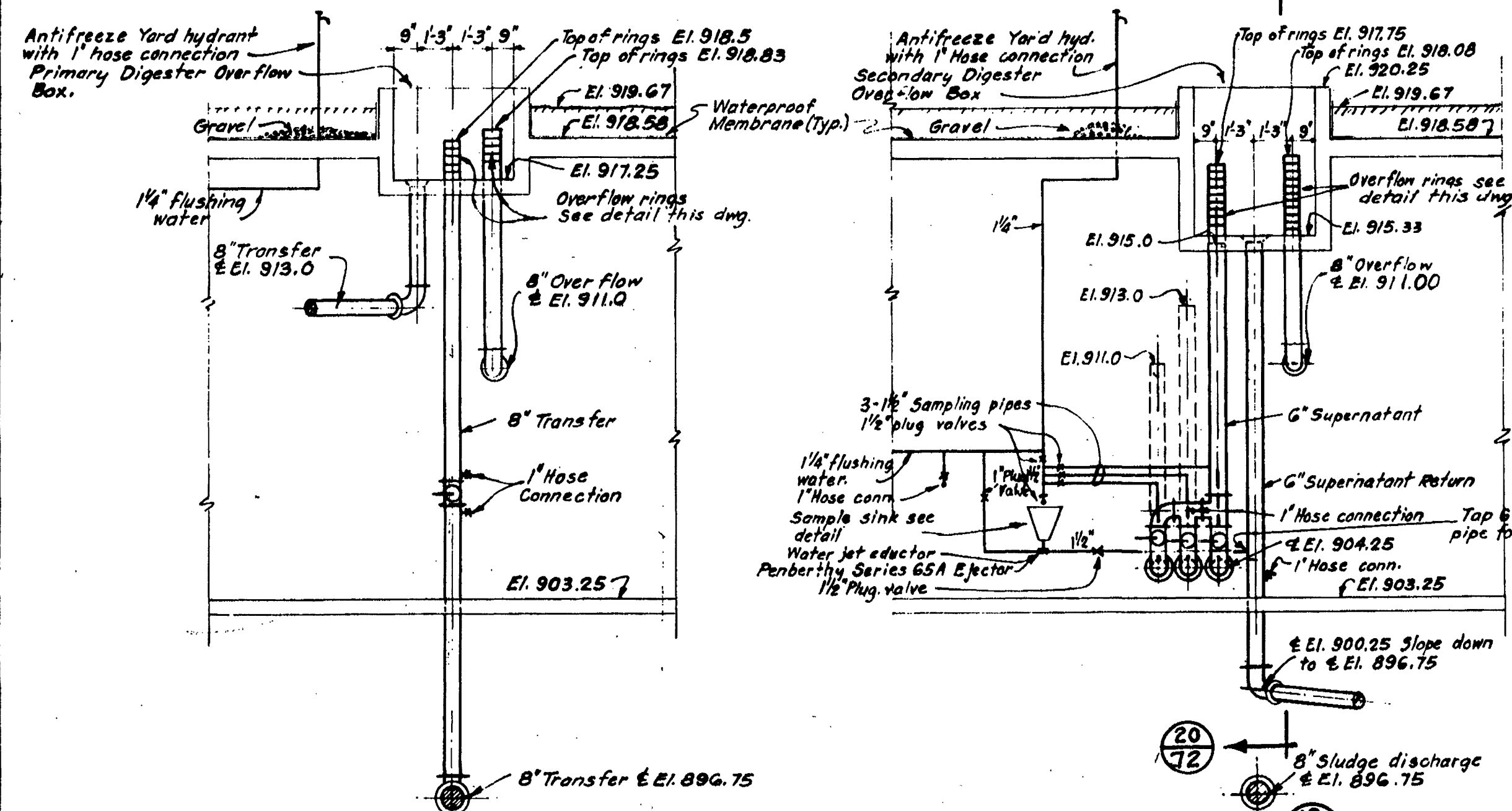
SECTION 18 Scale: 1/4" = 1'-0"
