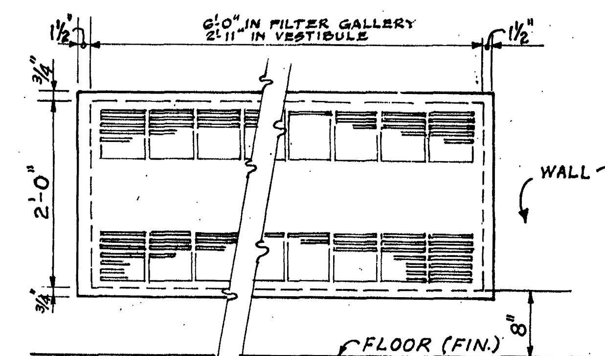
CONVECTOR GRILLE SCALE: 1" = 1'-0"
