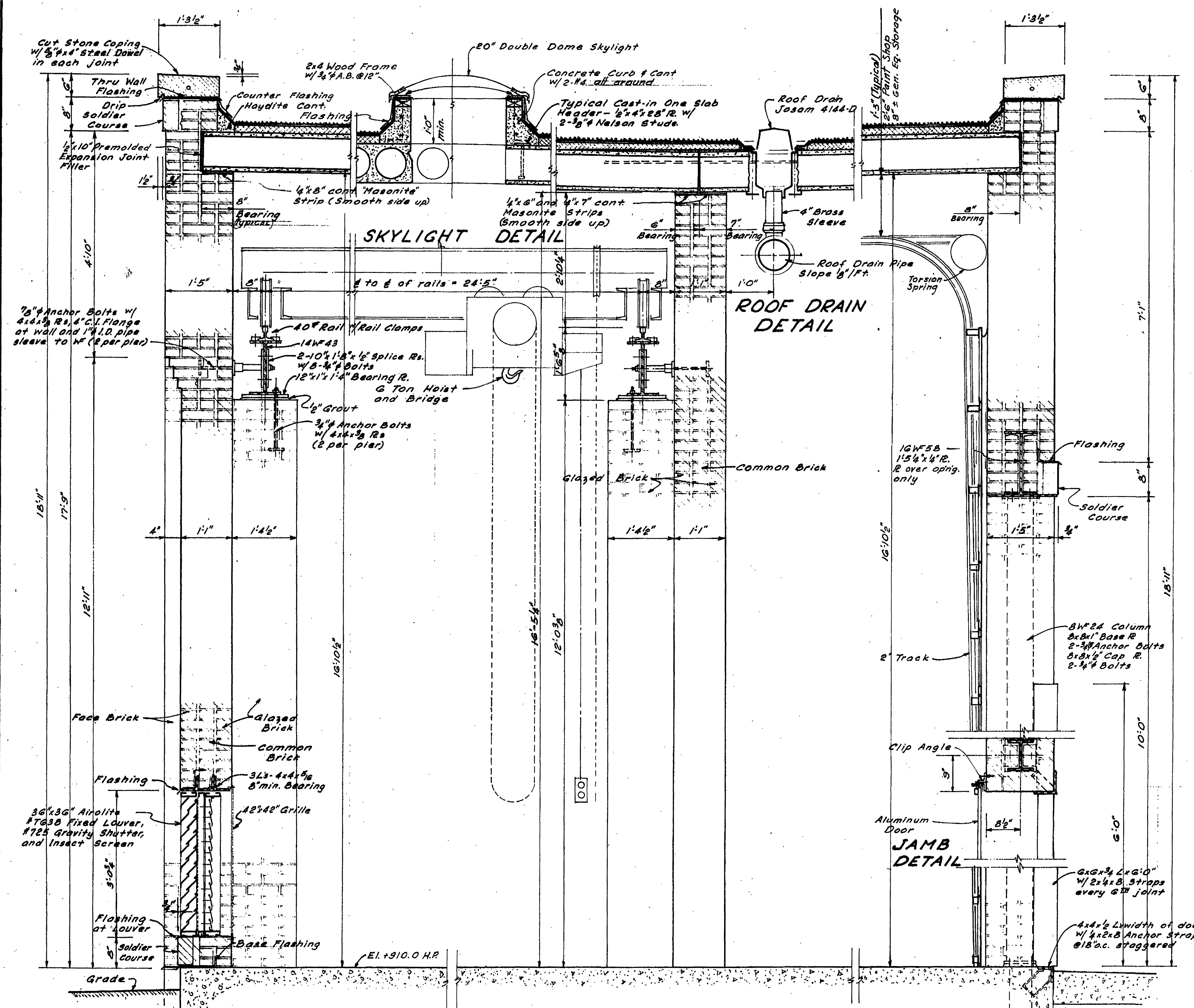
SECTION D Scale: 3/4"=1'-0"
