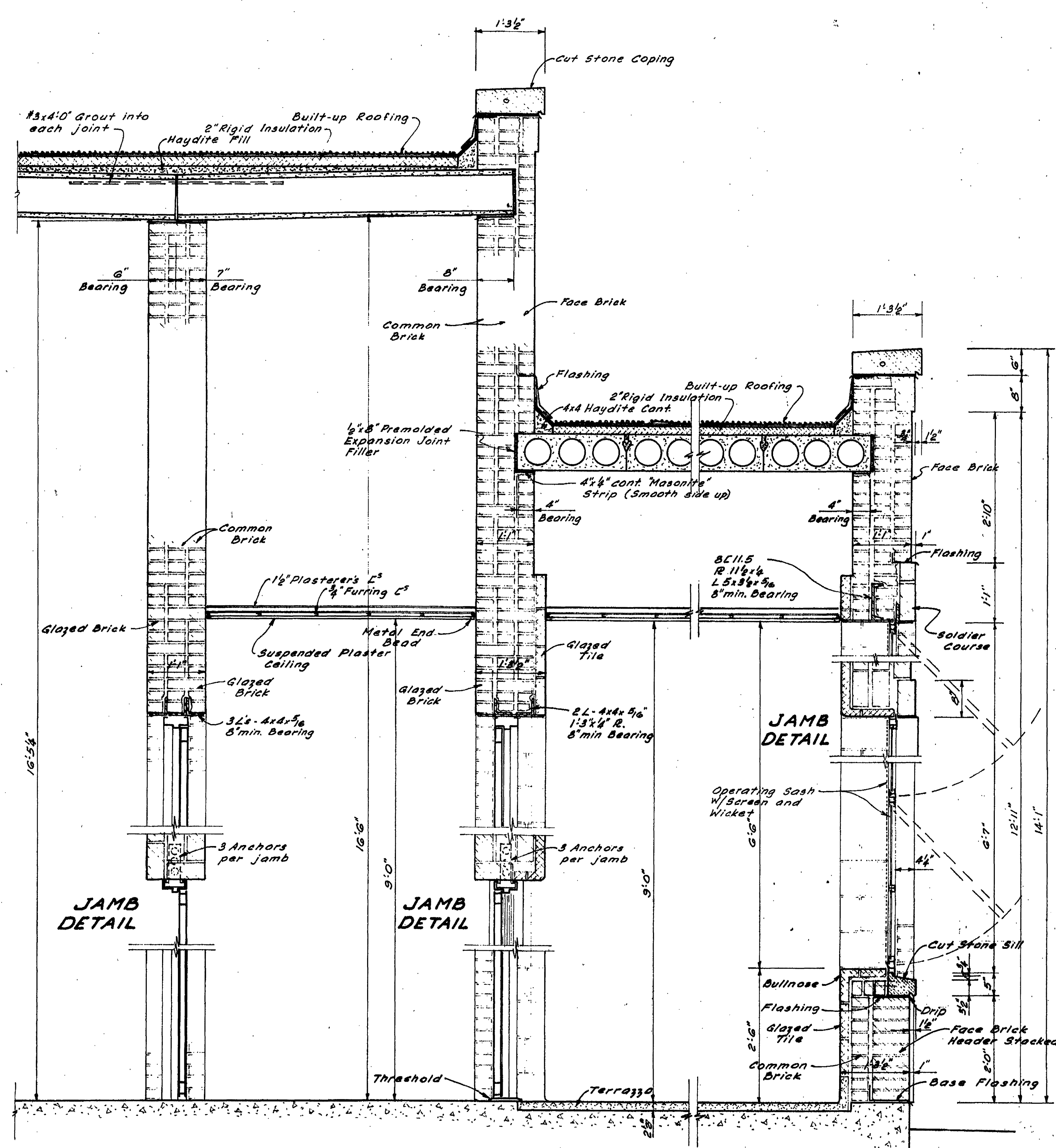
SECTION G Scale: 3/4"=1'-0"
