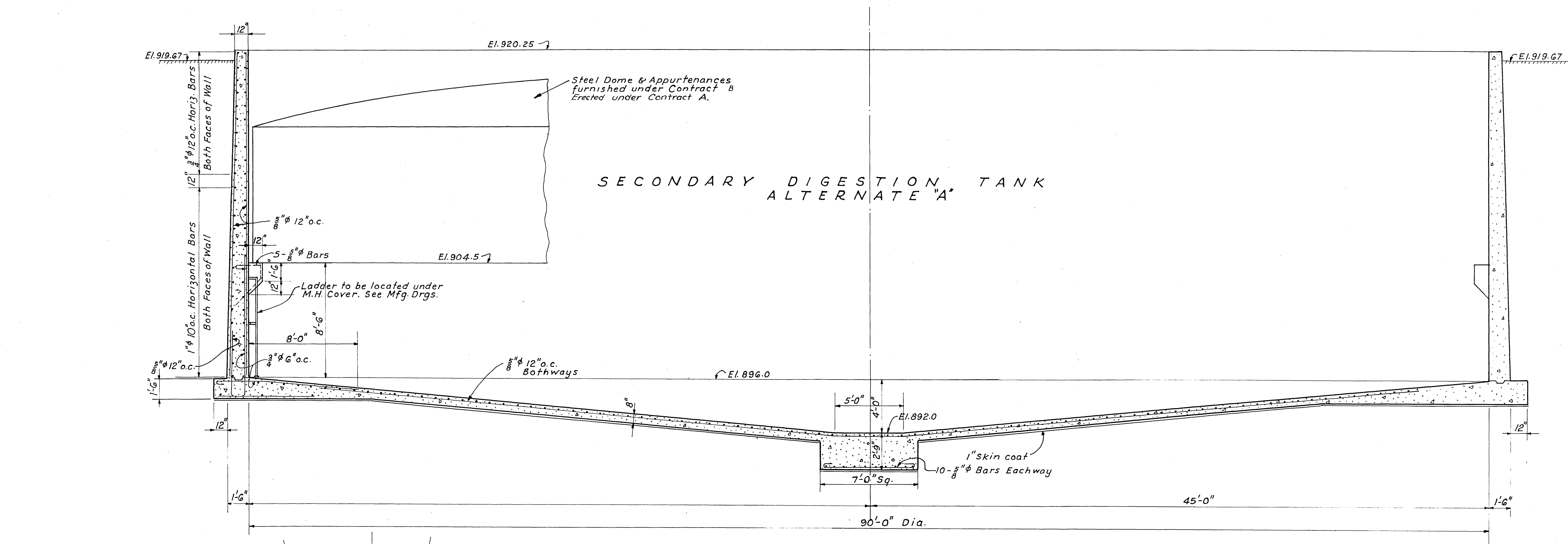
SECTION A-A Scale: \frac{1}{4}'' = 1'-0''
