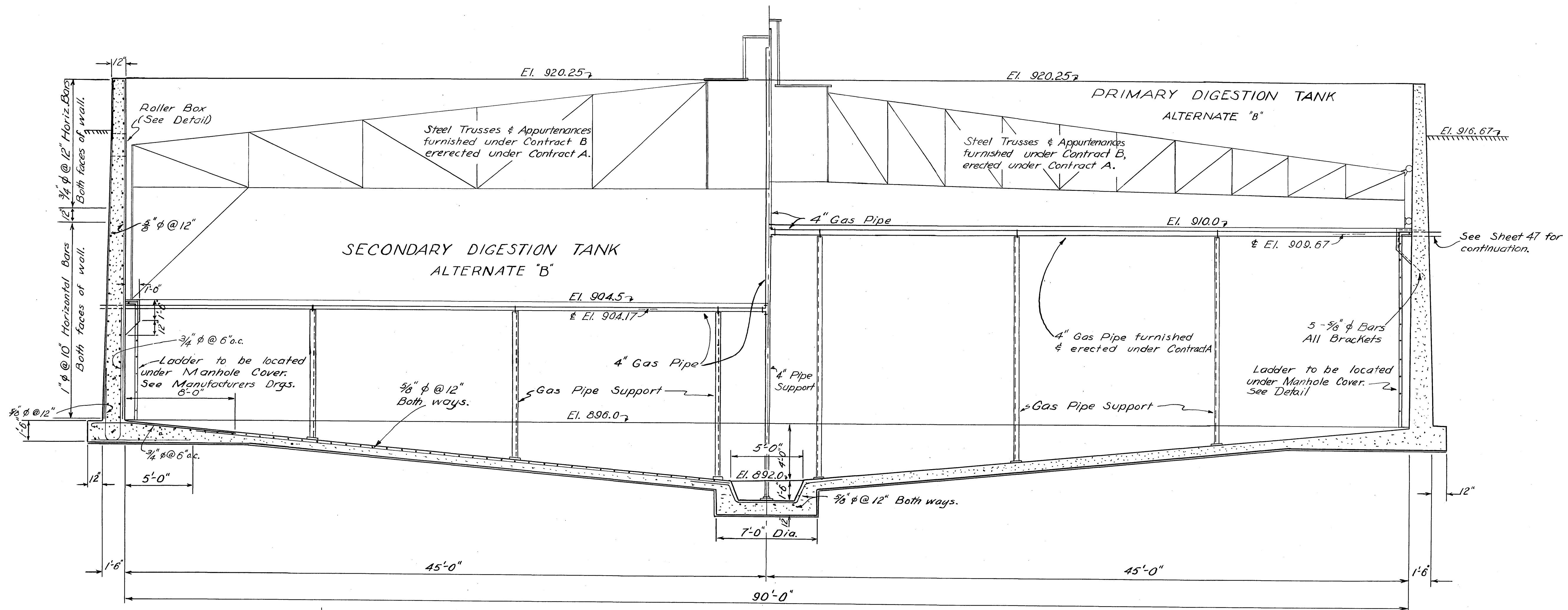
SECTION A-A Scale: 1/4" = 1'-0"
