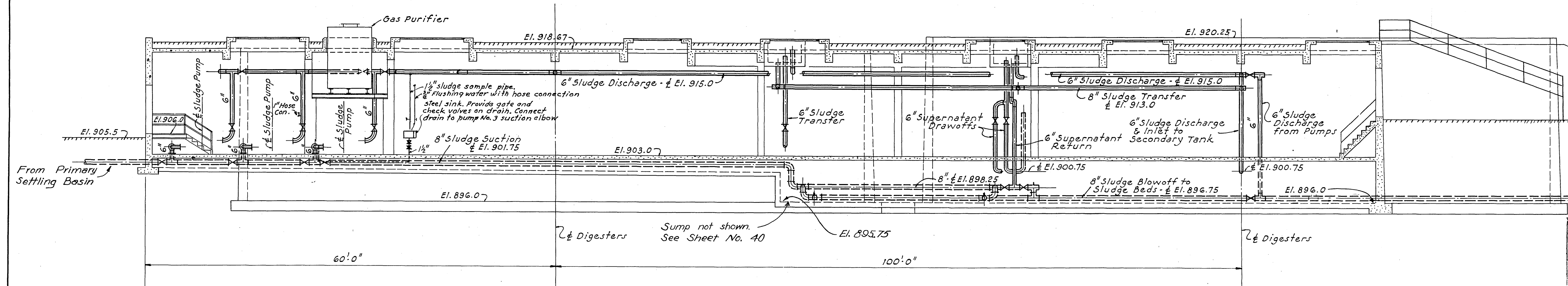
SECTION A-A SCALE: \frac{1}{8}" = 1'0"
