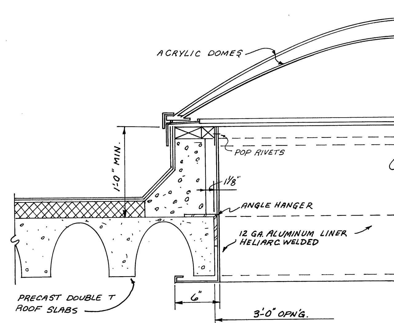
SKYLIGHT 10 7 SCALE: 1 1/2" = 1'-0"
