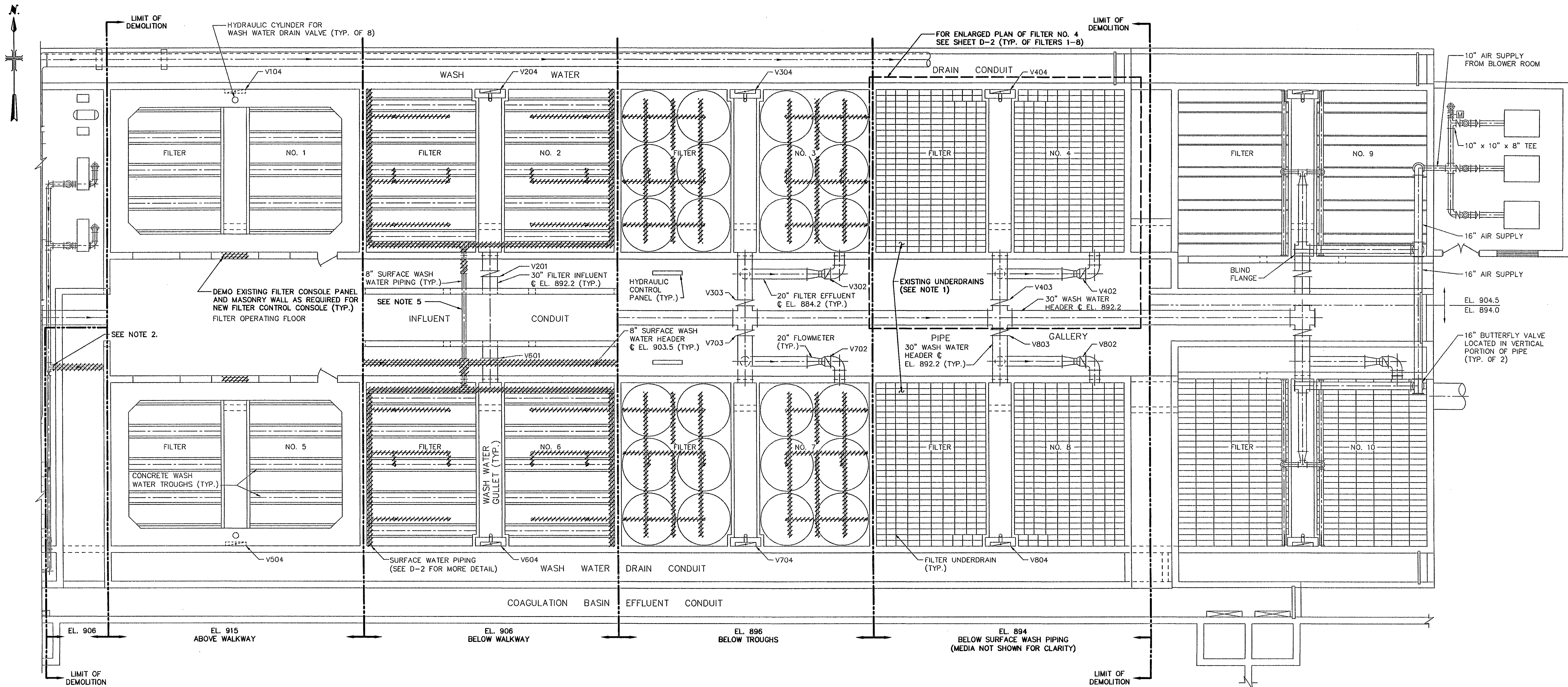
DEMOLITION PLAN SCALE: 1/8" = 1'-0"
