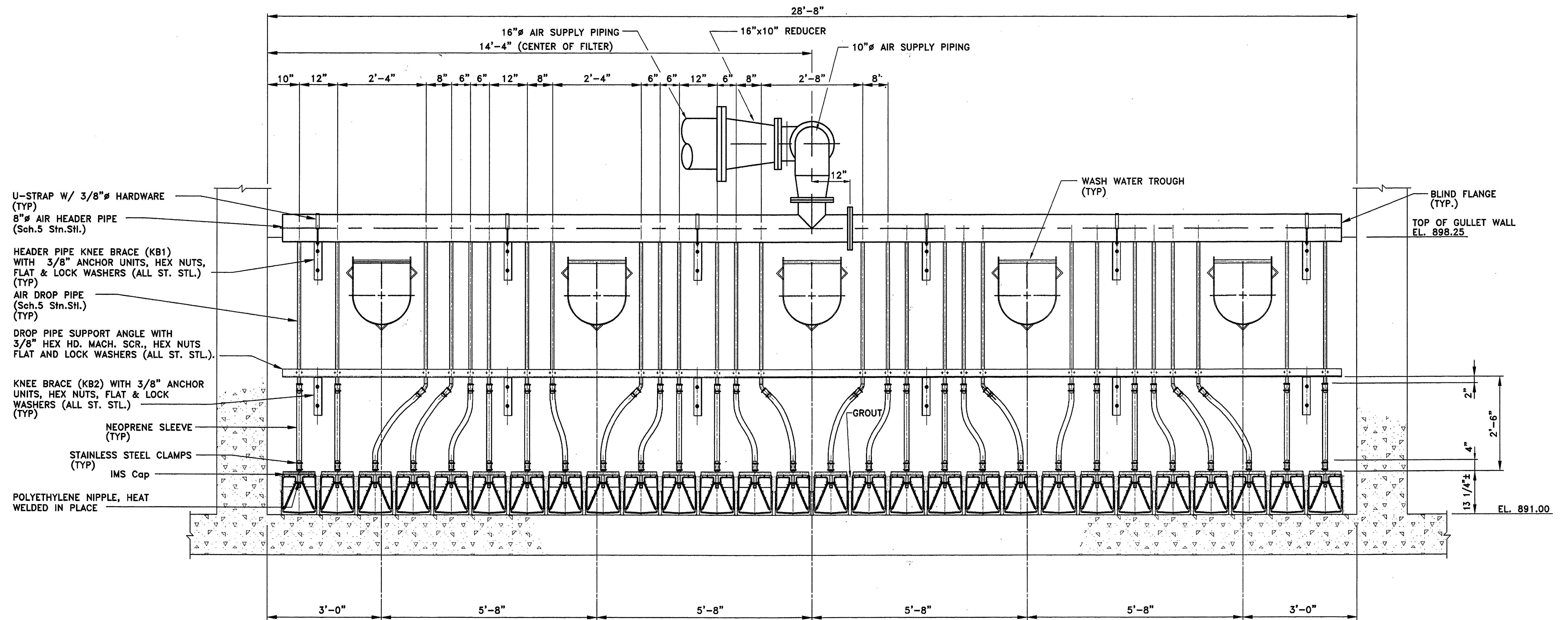
SECTION 3 SCALE: 3/4"=1'-0"
