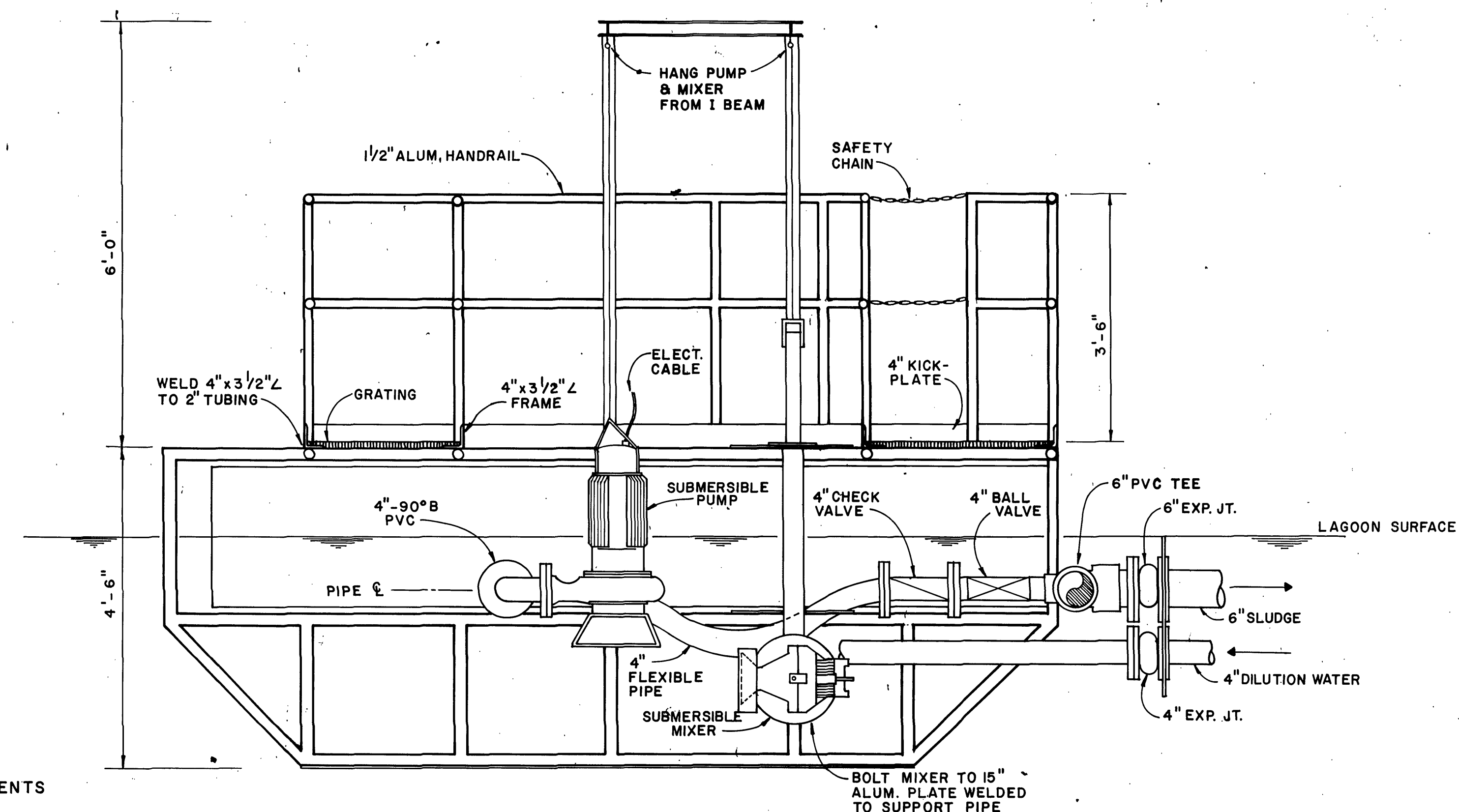
SECTION A-A SCALE: 3/4" = 1'-0"
