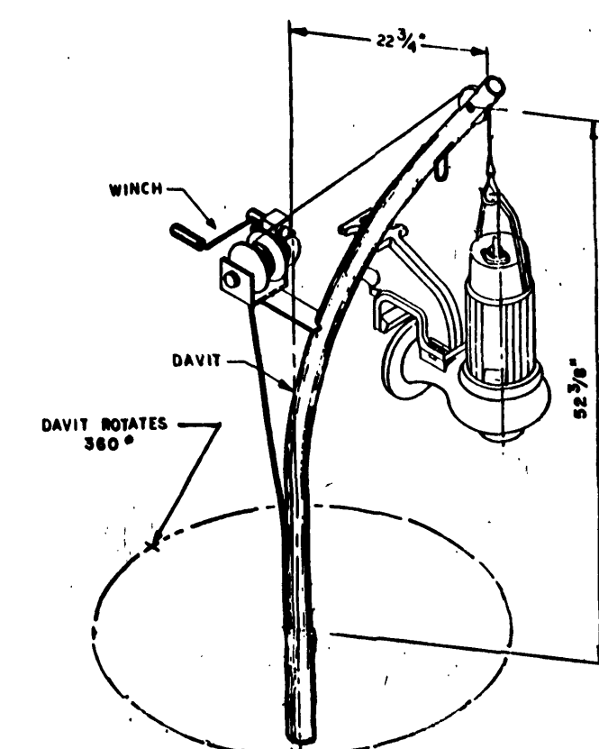
PORTABLE HOIST DETAIL N.T.S.
