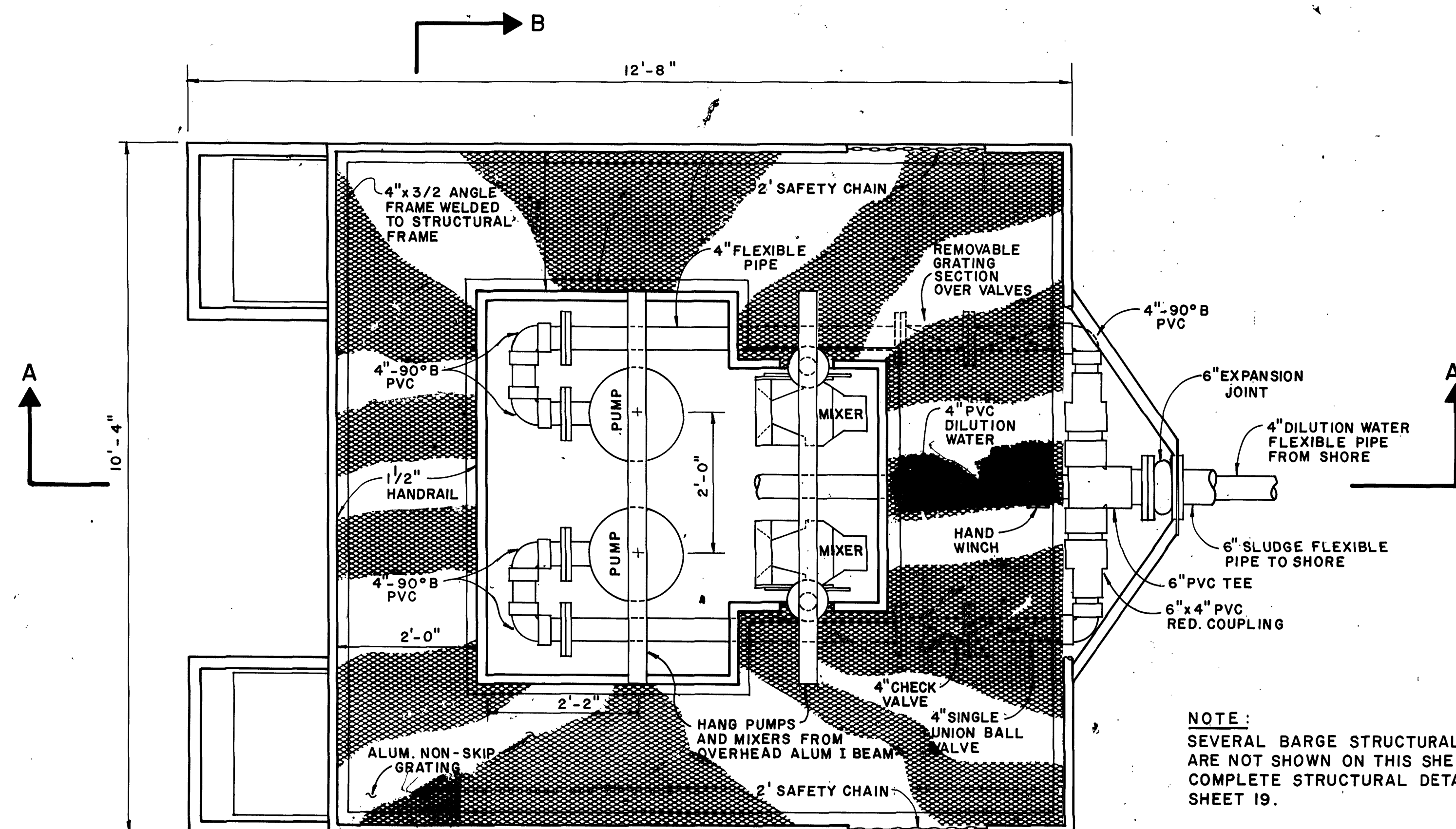
BARGE - PLAN SCALE: 3/4" = 1'-0"
